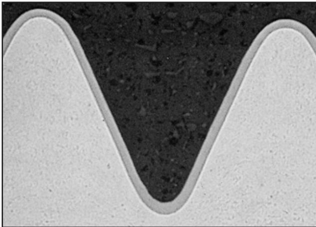
Bild 3 Beschichtetes Gewinde Figure 3 Coated thread
